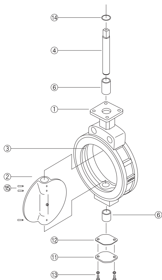
350A~600A本体図
