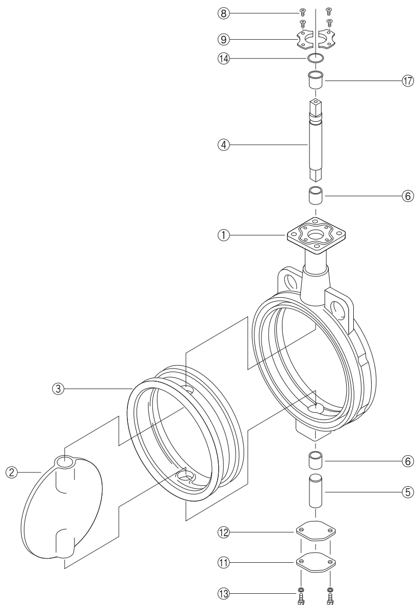
40A～300A本体図
